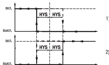
Рис. 7. Диаграммы срабатывания прибора по типам логики: 1 – обратное управление; 2 – прямое управление
