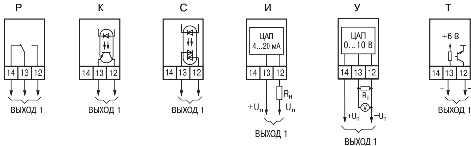
Рис. Б.2. Схемы подключения различных модификаций ВУ1
