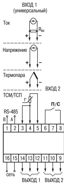
Рис. Б.1. Общая схема подключения
