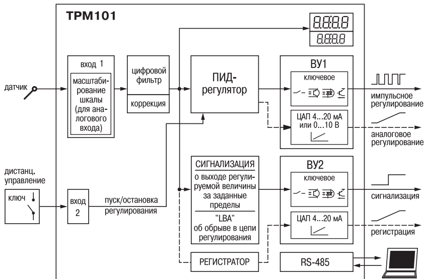
Рис. 2. Структурная схема TPM101
