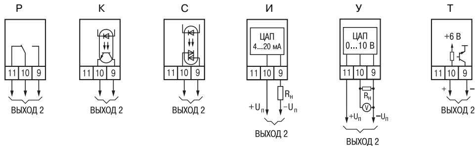
Рис. Б.3. Схемы подключения различных модификаций ВУ2
