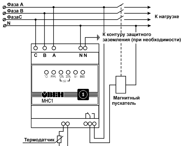
Рис. А. 1. Подключение прибора при работе в трехфазной сети
