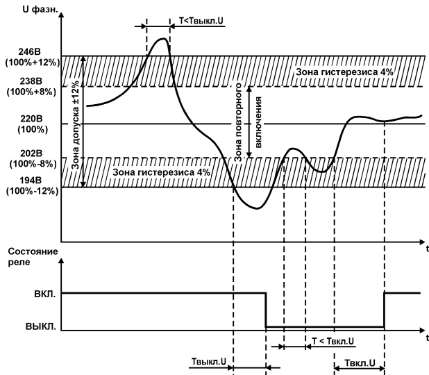
Рис. 3. Работа канала контроля напряжения при установленной зоне допуска в \pm 12\% и гистерезисе 4% от номинального в 220 В
