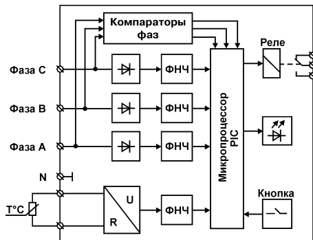
Рис. 2 Функциональная схема МНС1
