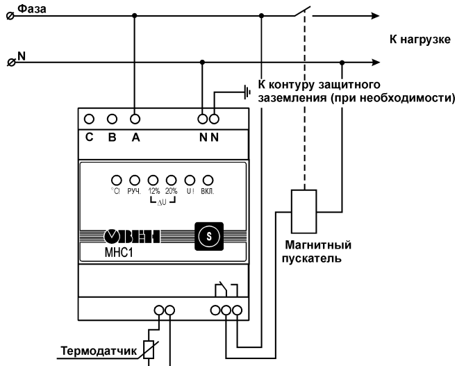
Рис. А.2. Подключение прибора при работе в однофазной сети
