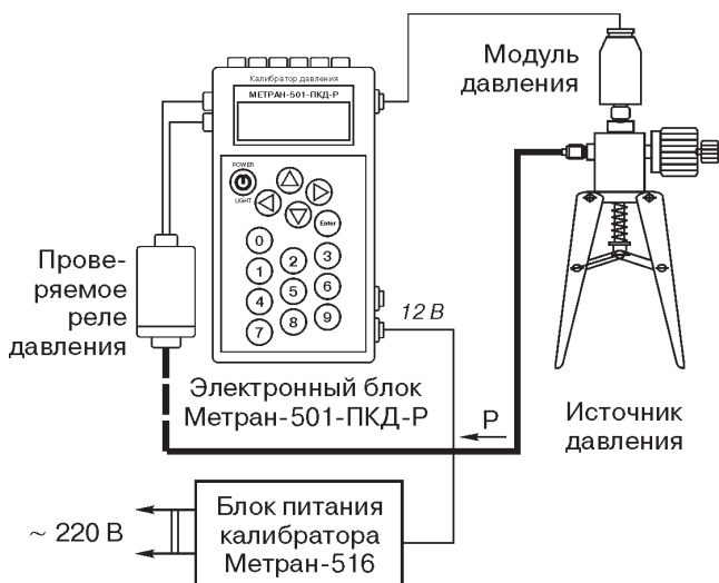
Рис. 6. Поверка и калибровка реле давления.
