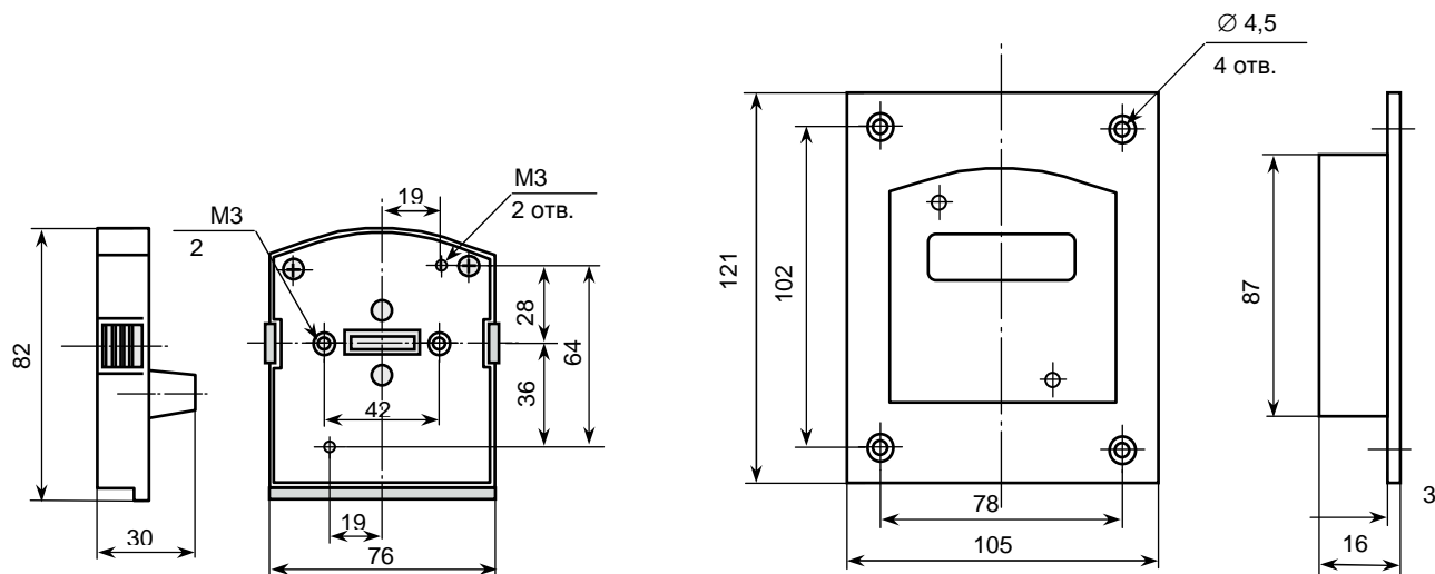
Монтажная рамка
