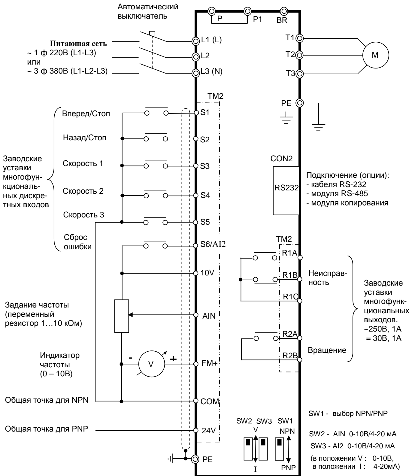
П2.1. Схема подключения силовых и управляющих цепей: моделей E2-8300-SP5L, -S1L, -S2L, -001H, -002H.
