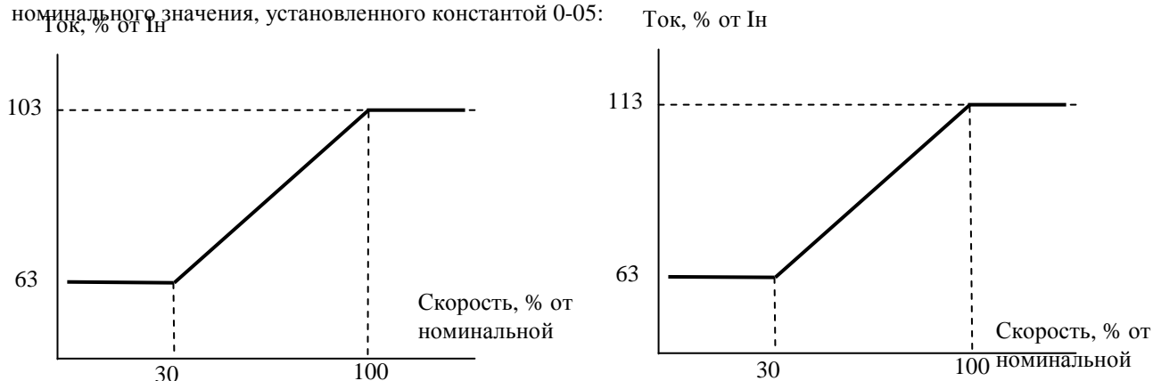
Нагрузка с постоянным моментом (9-10 = 0)
