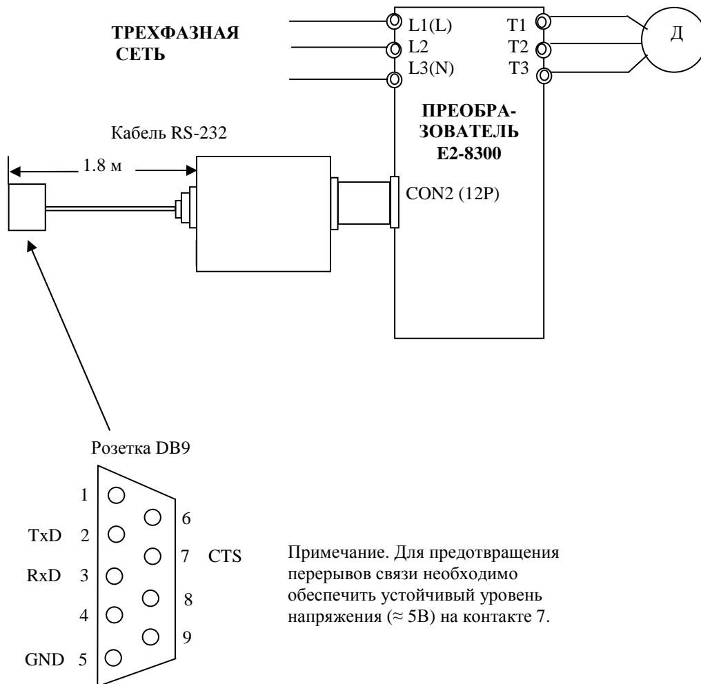
Схема подключения кабеля RS-232
